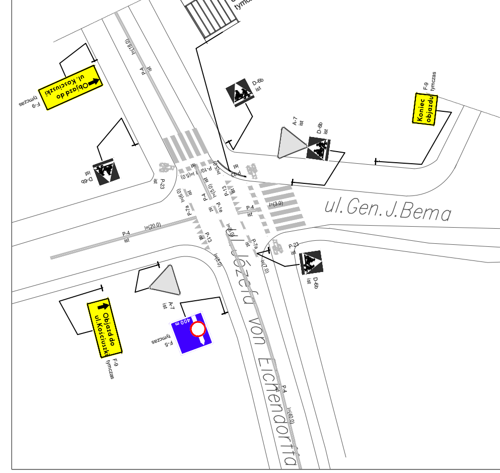
Oznakowanie skrzyżowania ul. J.von Eichendorfa/ ul. Gen.J. Bema/ ul.L.Waryńskiego
