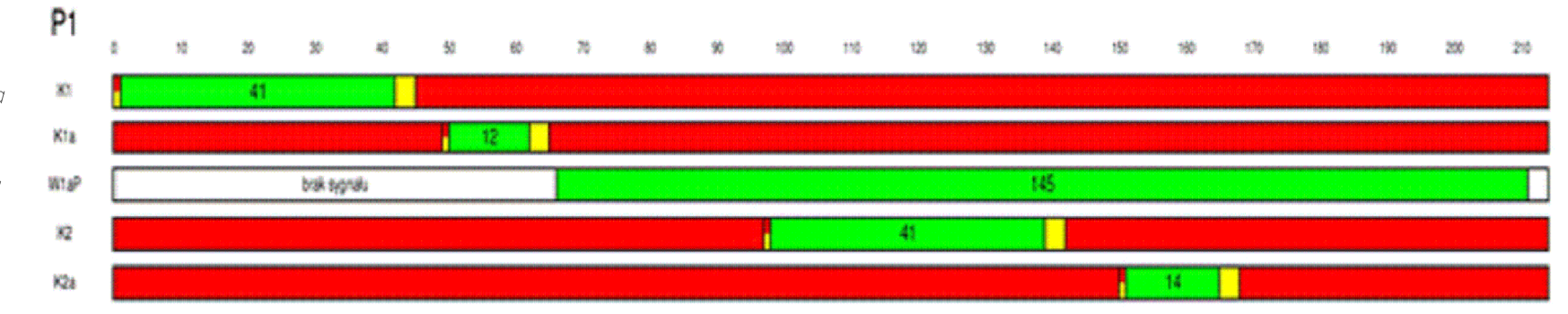
Program sygnalizacji wahadkowej
